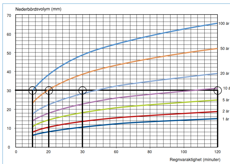
Nederbördsvolym som funktion av varaktighet och återkomsttid baserat på (Dahlström 2010), hämtad från Svenskt Vattens publikation P110.
