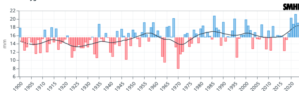
Maximal dygnsnederbörd i Götaland under vintern
